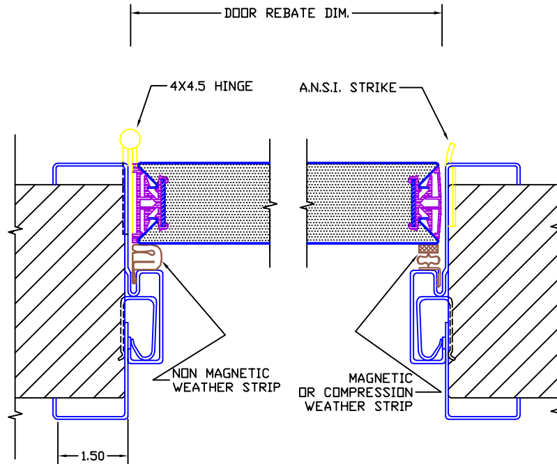
HINGE JAMB DETAIL
